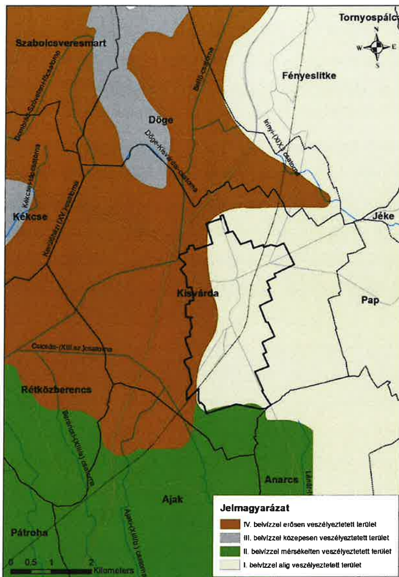
6. ábra Kisvárdai belvíz veszélyeztetettsége
